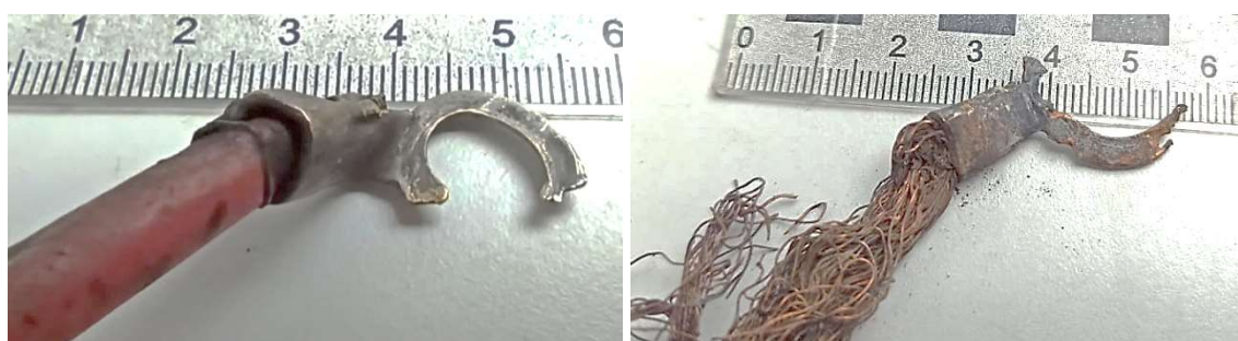
Рис.5. Локальные повреждения клемм, присоединяемых к стартеру
